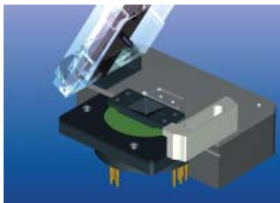
上面図 (マニュアルにて製品挿入) Upper view (Manually insertion)
